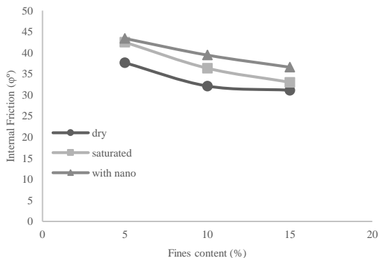
شکل (۱۷): تأثیر نانو سیلیس کلئیدی بر پارامترهای مقاومتی نمونه‌های خاکی مورد مطالعه
