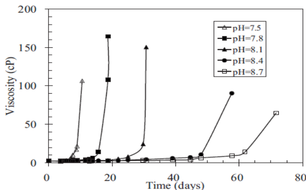
شکل (۲): تغییرات ویسکوزی‌تر در مقادیر مختلف PH برای محلول نانو سیلیس با ۵ درصد وزنی [۵]
