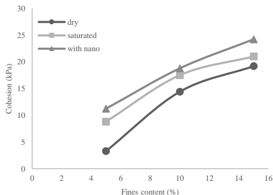
شکل (۱۷): تأثیر نانو سیلیس کلئیدی بر پارامترهای مقاومتی نمونه‌های خاکی مورد مطالعه
