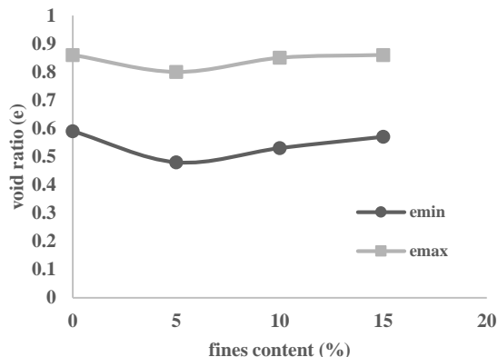
شکل (۶): تغییرات نسبت تخلخل حداقل و حداکثر در نمونه‌های مورد مطالعه
