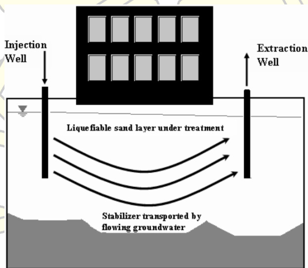
شکل (۱): مفهوم تثبیت غیر محرک [۲]
