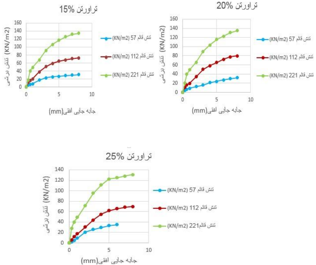
شکل ۱۱: نمودار تنش برشی - جا به جایی افقی برای ماسه خالص و مخلوط ماسه و گل سنگ تراورتن و گرانیت.
