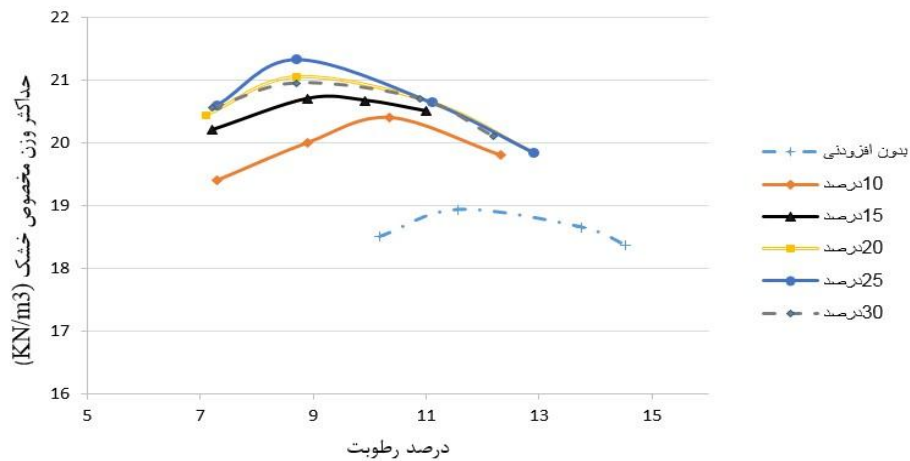
شکل ۳: منحنی تراکم ماسه - پودر سنگ گرانیته.
