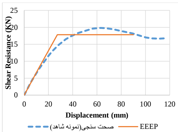
شکل ۱۳: منحنی دوطرفی (ASTM E2126-07).
