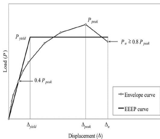
شکل ۱۴: منحنی دوطرفی صحت سنجی (نمونه شاهد).
