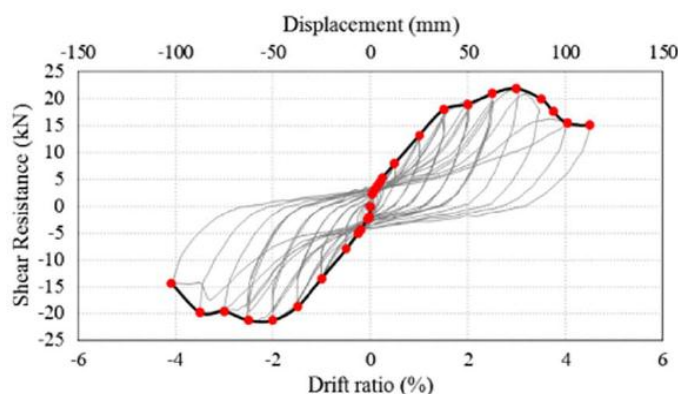
شکل ۲: منحنی بار-جابه‌جایی تحت بارگذاری سیکلیک نمونه آزمایشگاهی [۶].
