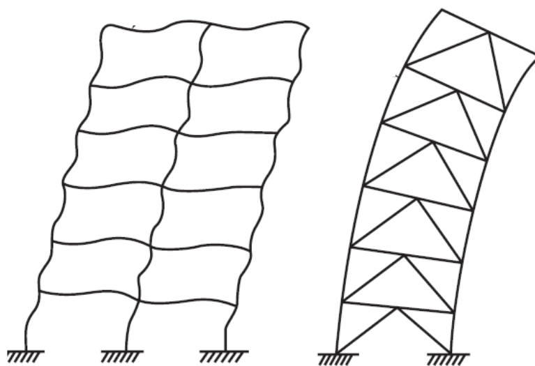
شکل ۴: تغییر شکل برشی و خمشی [۶].
