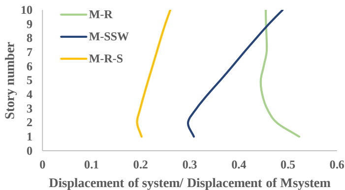
شکل (۱۴): نسبت تغییر مکان سامانه ها، مدل ۱۰ طبقه.
