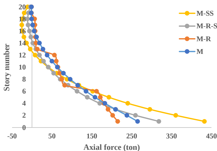
شکل (۱۸): حدکثر نیروی محوری در ستون برای سازه‌های ۲۰ طبقه.
