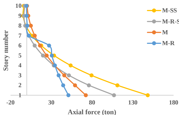
شکل ۱۷: حدکثر نیروی محوری در ستون برای سازه‌های ۱۰ طبقه.
