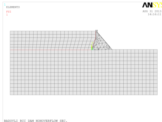
شکل ۸: مدل اجزاء محدود برای بلندترین مقطع غیرسرریز.
