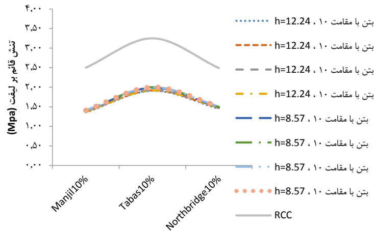
شکل ۲۷: ماکزیمم تنشهای قائم بر لیفت (MPa) در مدل‌های مطرح شده در مقطع غیرسرریز متناظر سطح زلزله MCE.
